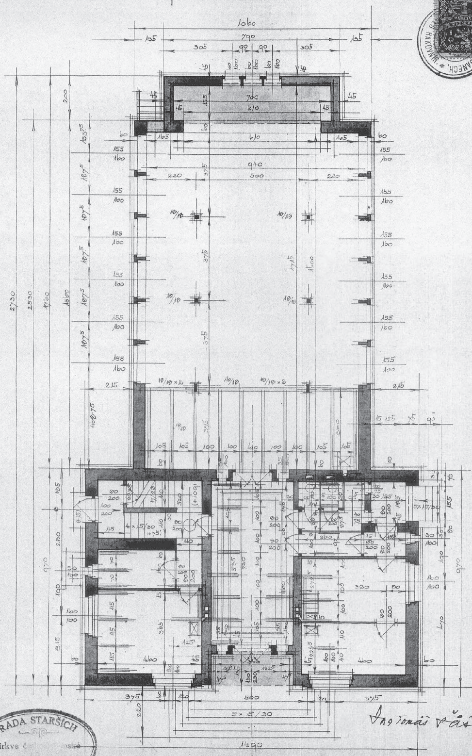
Přídorys přízemí (OÚ Lužná)
