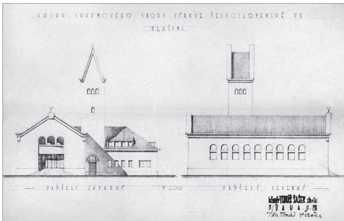
Nezrealizovaný plán sakrálního objektu ve Vlašimi (ÚAM CČSH Praha)
